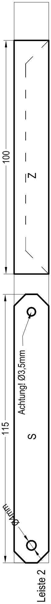
Plan 7 Leiste 1
